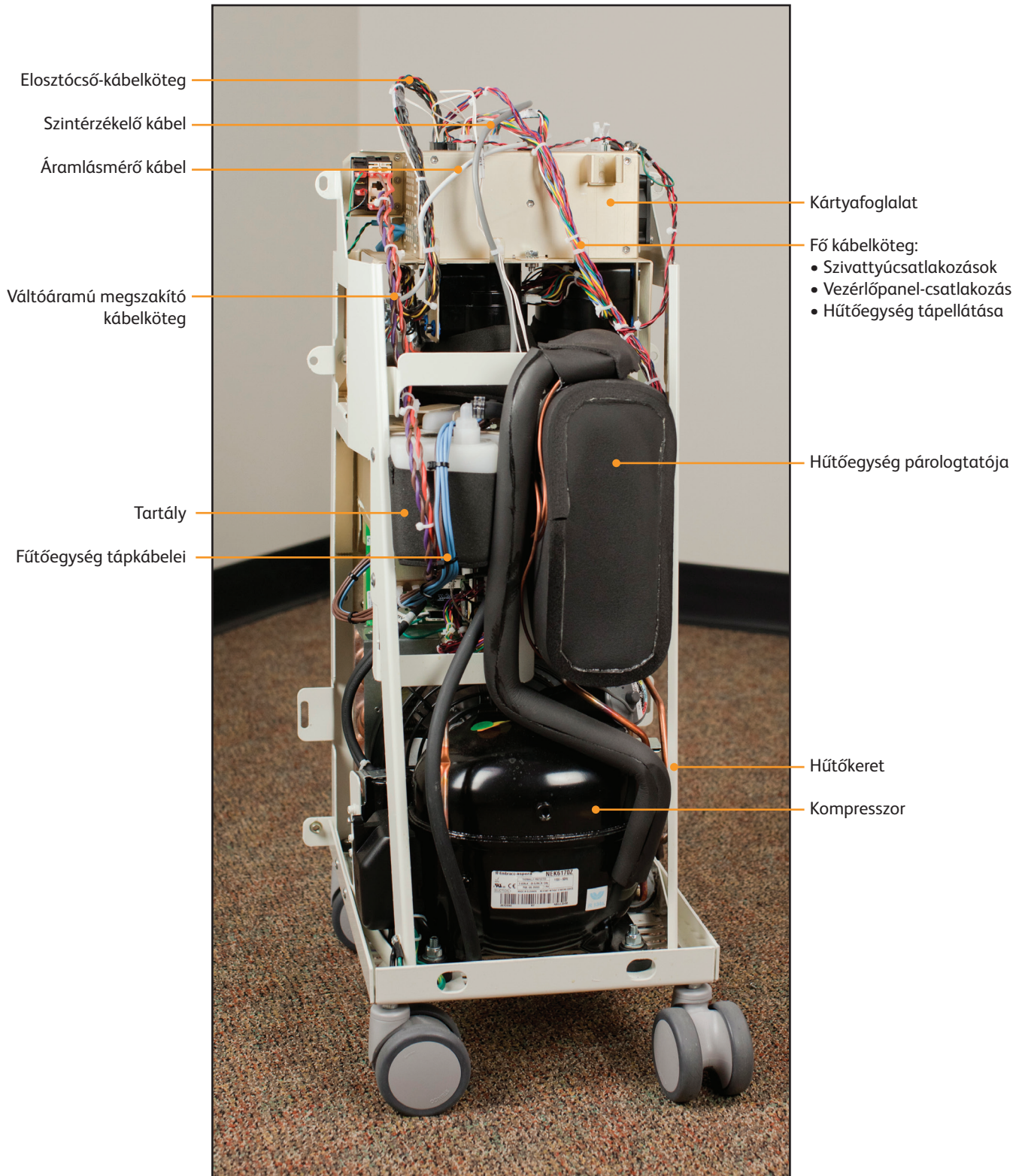
8-2. ábra Vezérlőmodul, előlső belső nézet
