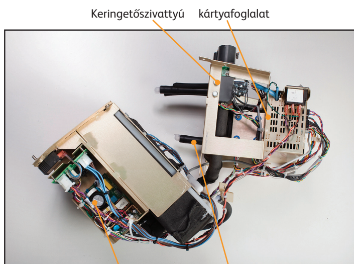
Keringetőszivattyú keverőszivattyú Fűtőegység szintérzékelő kártyafoglalat
