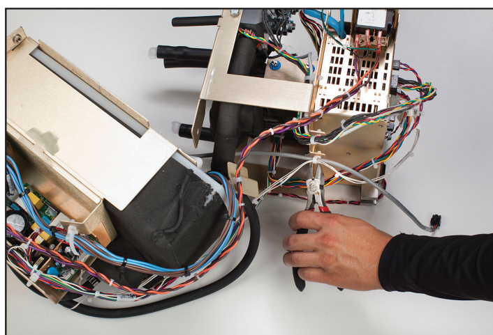
8-27. ábra Vágja el a kábelkötegelőket (3. lépés)
