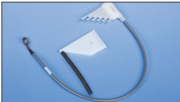
8-64. ábra Szintérzékelő
