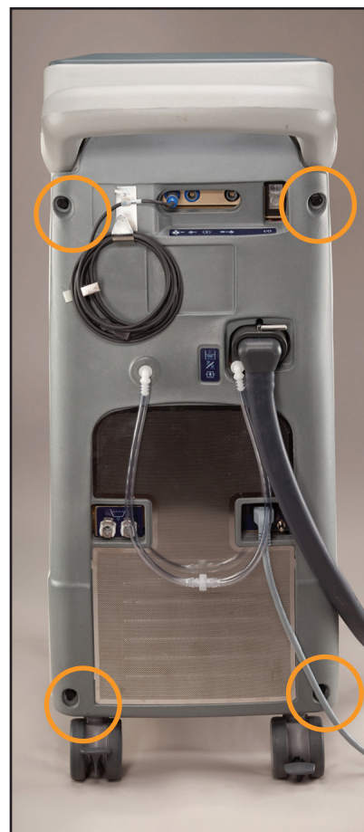
8-10. ábra Hátsó panel megjelölt eltávolítandó csavarokkal (2. lépés, balra)
