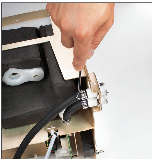
8-43. ábra Nyissa ki a bilincset, amely a hűtőszivattyút a leeresztőszelephez rögzíti
