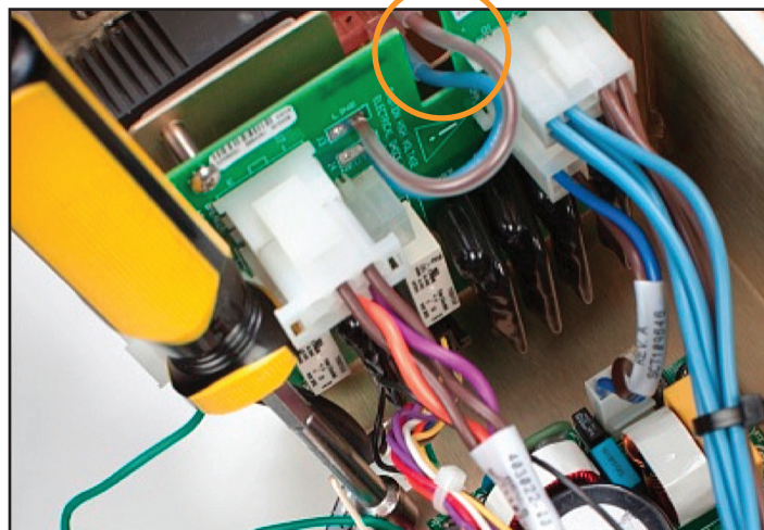
Afb. 8-69 Netspanningscircuitkaart in positie, met aansluitingen op hun plaats
