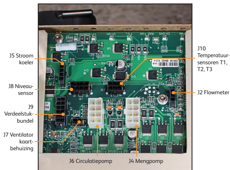
Afb. 8-15 Aansluitingen I/O-circuitkaart
