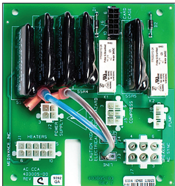
Afb. 8-68 Netspanningscircuitkaart
