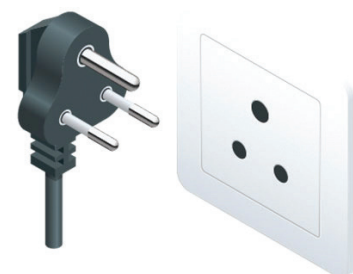
Voedingskabel 733-08 Type M - Zuid-Afrika
