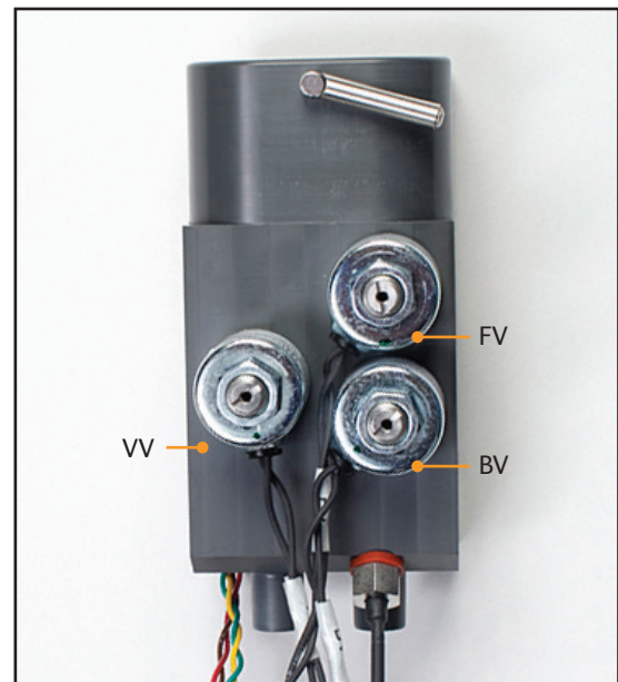
Afb. 8-62 Verdeelstuk, weergave van de positie van de 3 solenoiden (stap 8)
