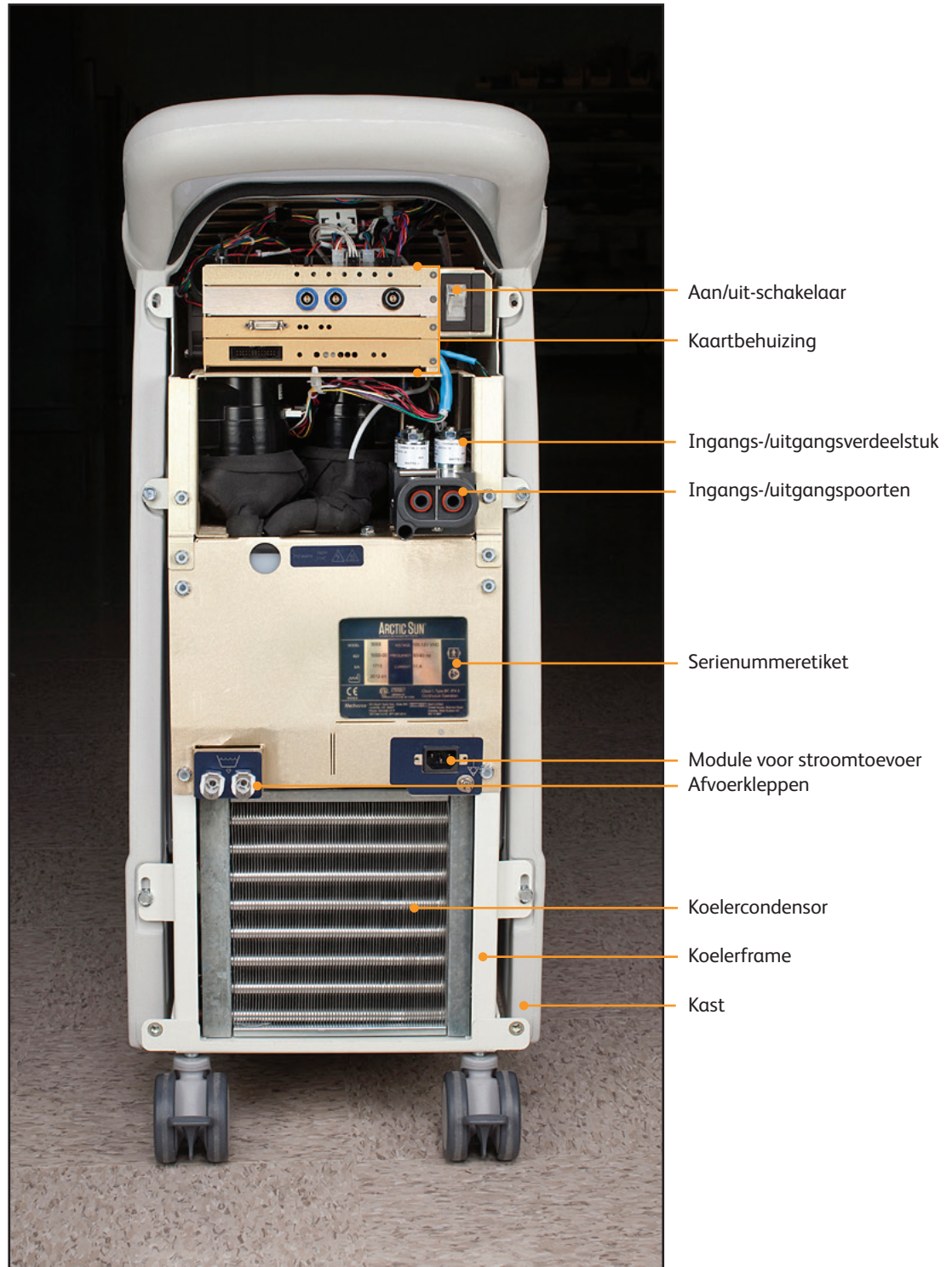
Afb. 8-1 Controlemodule, achteraanzicht na verwijdering van achterpaneel
