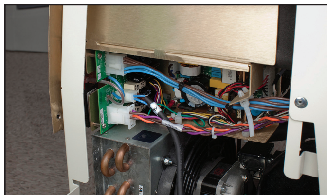
Afb. 8-20 Koppel de grijze kabel van de stroomaansluiting van de koeler los; locatie aangegeven (stap 2)
