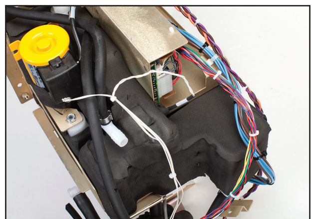
Afb. 8-58 Draadbundel tanktemperatuursensoren op zijn plaats
