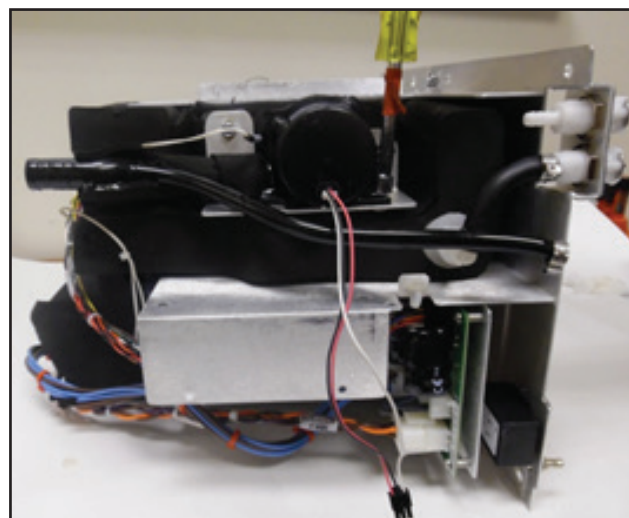
Afb. 8-46 Bouten verwijderen (stap 4)
