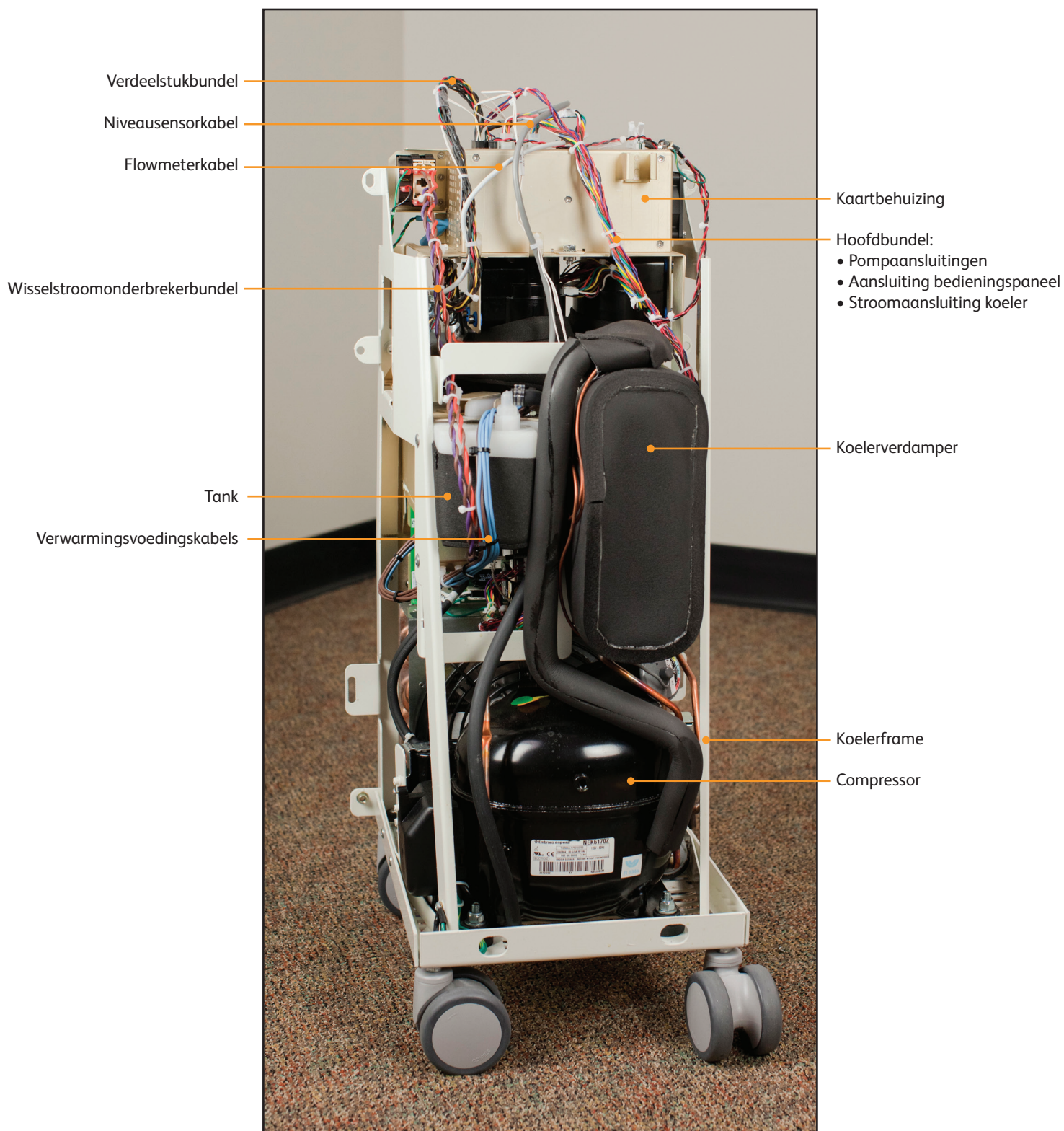
Afb. 8-2 Controlemodule, vooraanzicht binnenzijde
