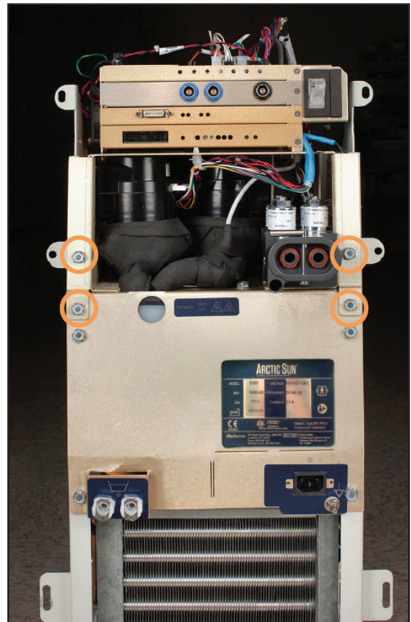
Afb. 8-16 Verwijder vier bouten (stap 1)
