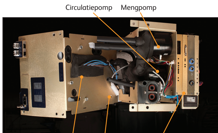
Verwarming Niveausensor Kaartbehuizing
