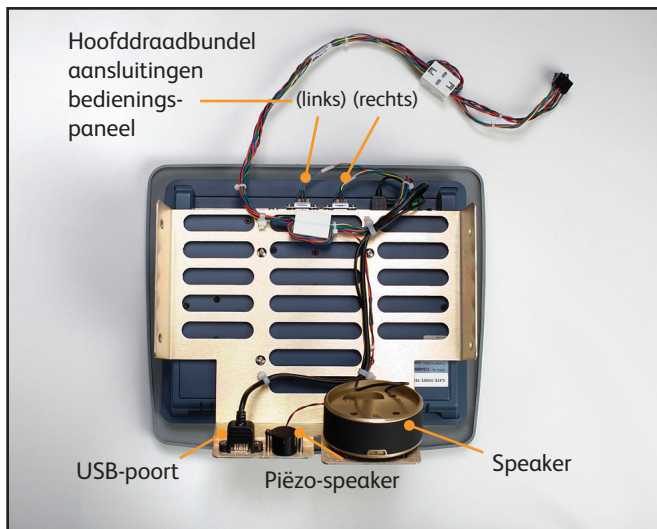
Afb. 8-55 Bedieningspaneel (achteraanzicht)
