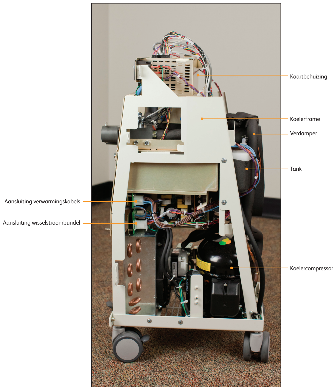
Afb. 8-4 Controlemodule, linkeraanzicht binnenzijde
