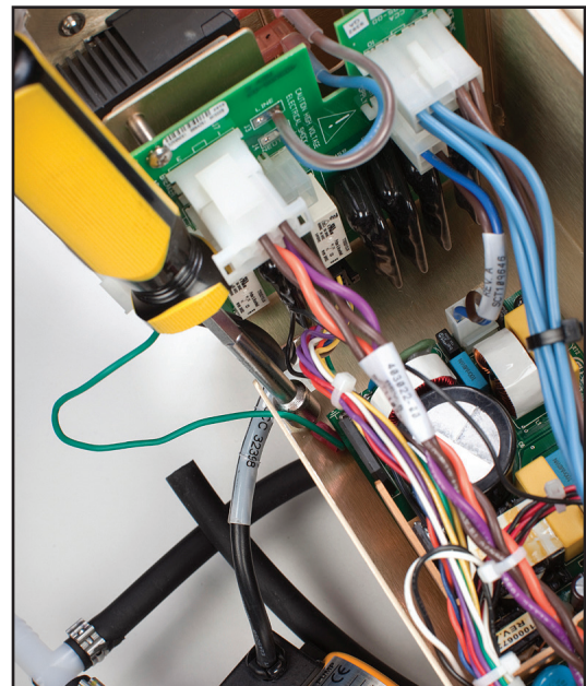
Afb. 8-40 Te verwijderen aardverbinding; locatie van moer is aangegeven (stap 3)
